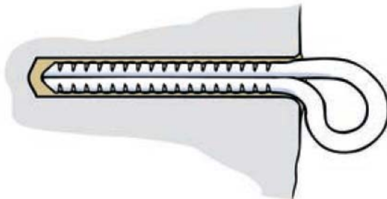
Abb. 1 Verbundanker, -haken
