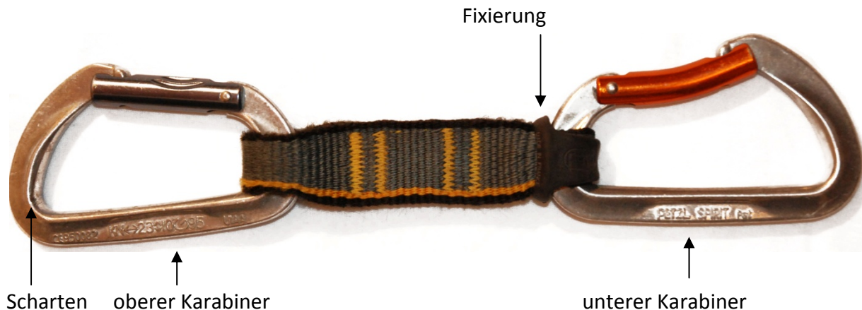
Abb. 6 Expressschlinge
